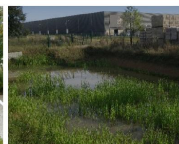
Ouvrage de gestion des eaux pluviales
